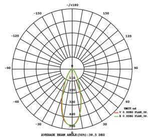
3.5W Module
